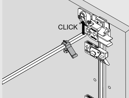
Insert synchronisation linkage
